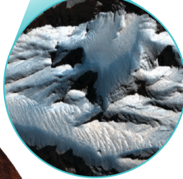
Fotografía Tomada por el instrumento HIRISE de la sonda Mars en la zona de Tithonium Chasma, una parte de Valles Marineris.
